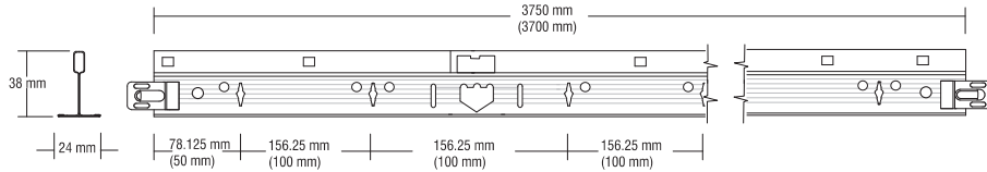
Tragschiene
