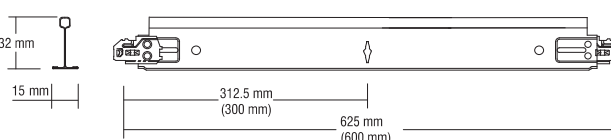
Kurze Querschiene
