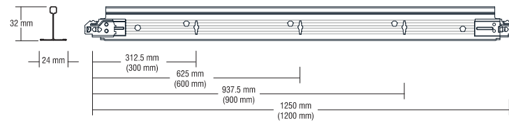
Kurze Querschiene
