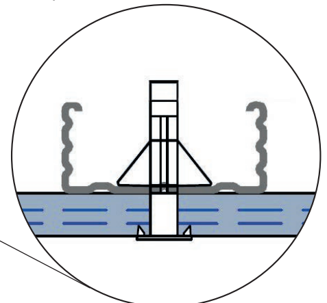
Detailansicht (Schnitt links um 90° gedreht) Lage der Dübelkrallen parallel zu Kapillaren / 90° zum Mattenstamm!
