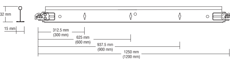
Kurze Querschiene
