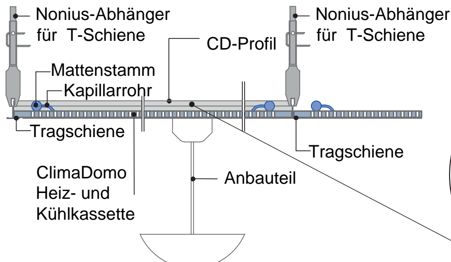
Detailansicht (Schnitt links um 90° gedreht) Lage der Dübelkrallen parallel zu Kapillaren / 90° zum Mattenstamm!
