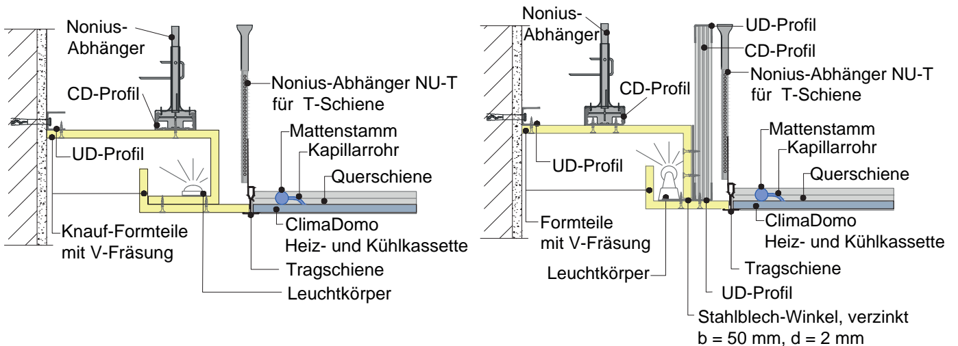
Auskragung mit GK-Formteil
